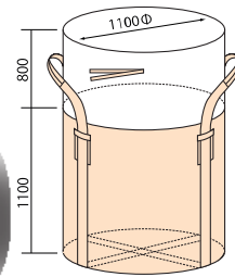
丸型スタンダードタイプ 反転ベルト：なし・あり
