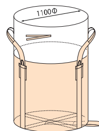
丸型スタンダードタイプ 反転ベルト：なし・あり
