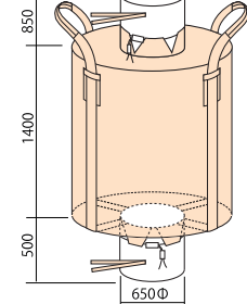
丸型・注入口・排出口半開
