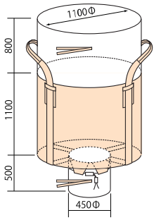
丸型・排出口半開
