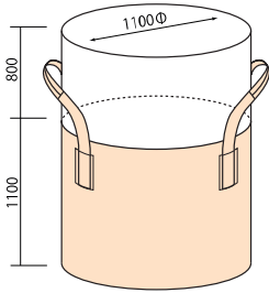
丸型・軽量物タイプ
