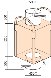
角型・注入口・排出口半開 2点吊り
