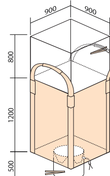
角型・排出口半開 2点吊り
