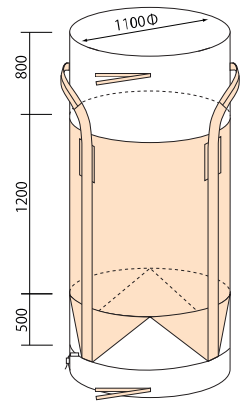
丸型・注入口・排出口全開
