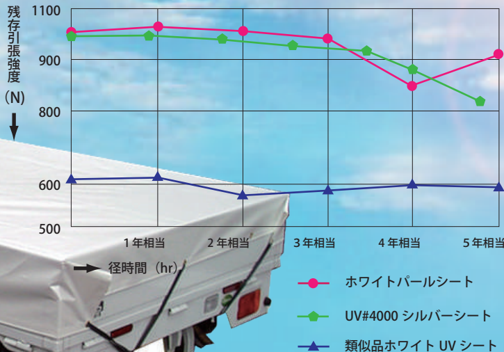
ホワイトパールシート残存強度比較
